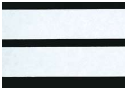
Prueba de adherencia con SEFAR® PET 1500: No hay residuos de partes de la pantalla en las bandas adhesivas, lo cual corrobora las excelentes propiedades de adherencia de SEFAR® PET 1500
