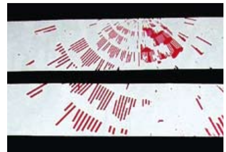
Prueba de adherencia con tejido de alto módulo sin tratamiento especial
